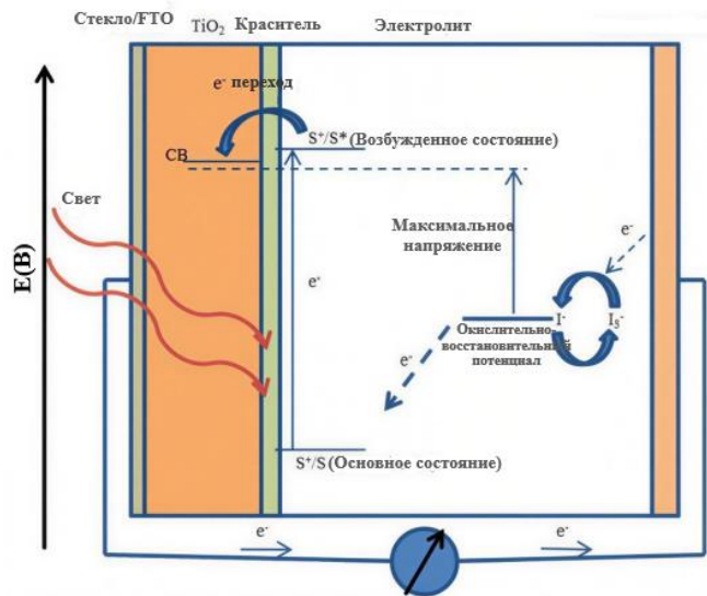
Рисунок 1.5 – Схема работы DSSC [14]
