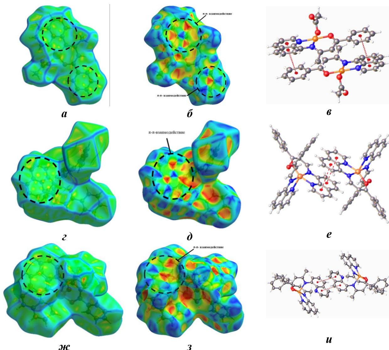
Рисунок 3.10 – Кривизна ( а, г, ж ), индекс формы ( б, д, з ) поверхности Хиршфельда и \pi - \pi - взаимодействие ( в, е, и ) комплексов 5 , 6 и 7
