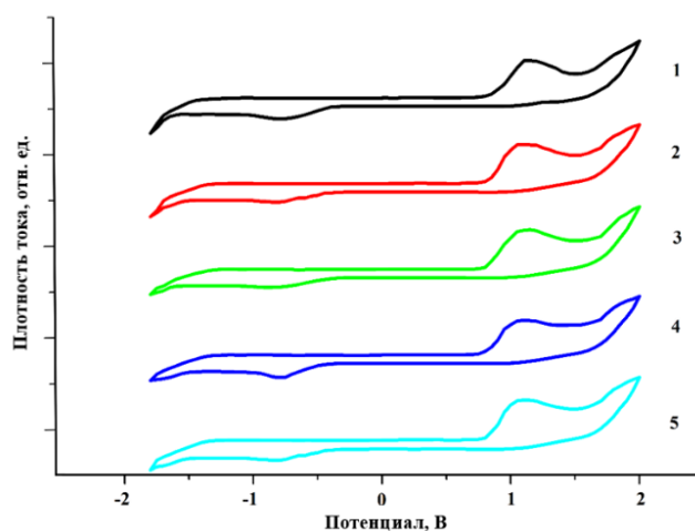
Рисунок 4.13 – Циклическая вольтамперометрия для комплексов 11а (1), 11б (2), 11в (3), 11г (4), 11д (5).
