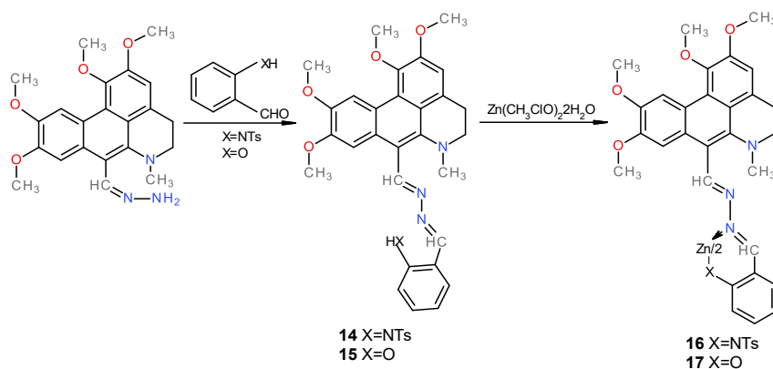
Схема 2.3 – Синтез хелатов цинка 16, 17 оснований Шиффа производных глутцина 14,15
