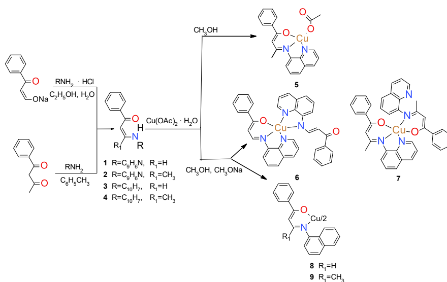
Схема 2.1 – Синтез хелатов меди 5 - 9 на основе \beta -аминовинилкетонов 1 - 4
