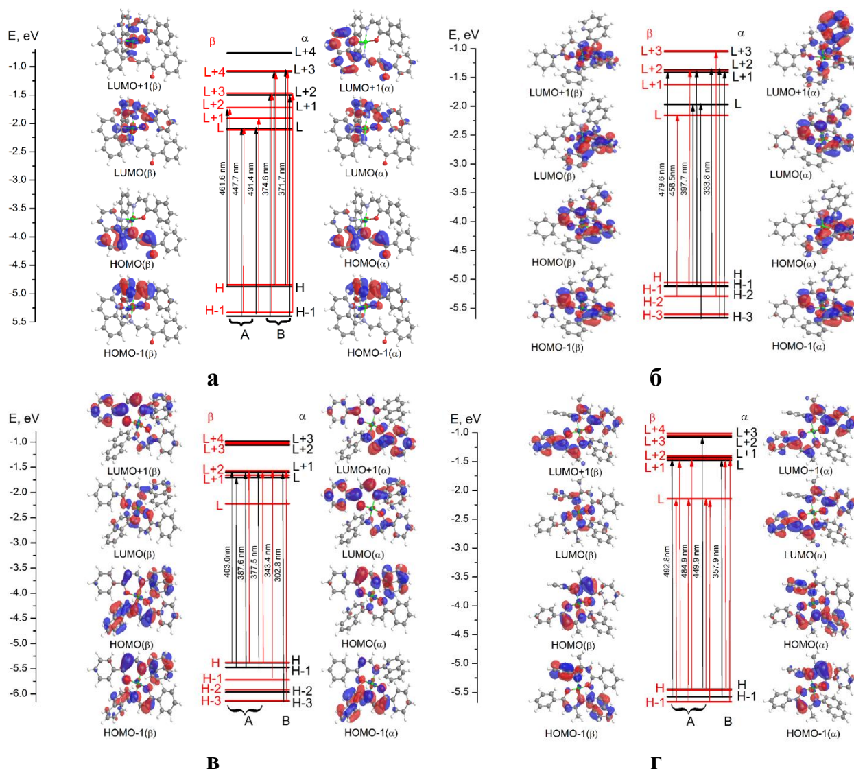
Рисунок 3.14 – Диаграмма энергетических уровней и изоповерхности пограничных молекулярных орбиталей комплекса 6 (а), 7 (б), 8 (в) и 9 (г) и основных орбитальных электронных переходов.
