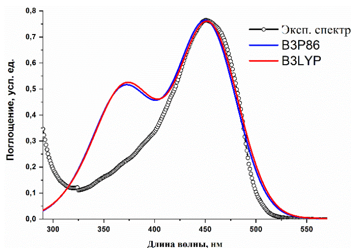
Рисунок 2.6 – Электронные спектры поглощения \beta -аминовинилкетонов меди(II)
