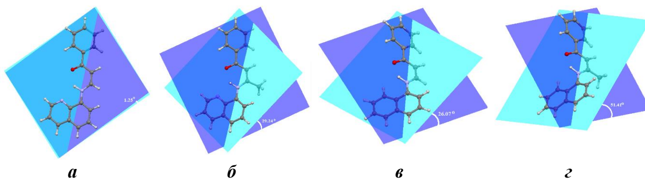
Рисунок 3.1 – Оптимизированные структуры 1 (a), 2 (б), 3 (в), и 4 (г)
