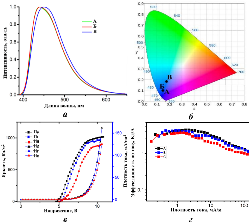
Рисунок 4.17 –Спектры электролюминесценции комплексов 11в - 11д в OLED А-В (а); Цветовая диаграмма CIE для устройств А-В (б). Вольт-яркостные и вольт-амперные характеристики устройств OLED А-В (в). График зависимости эффективности по току от плотности тока (г).
