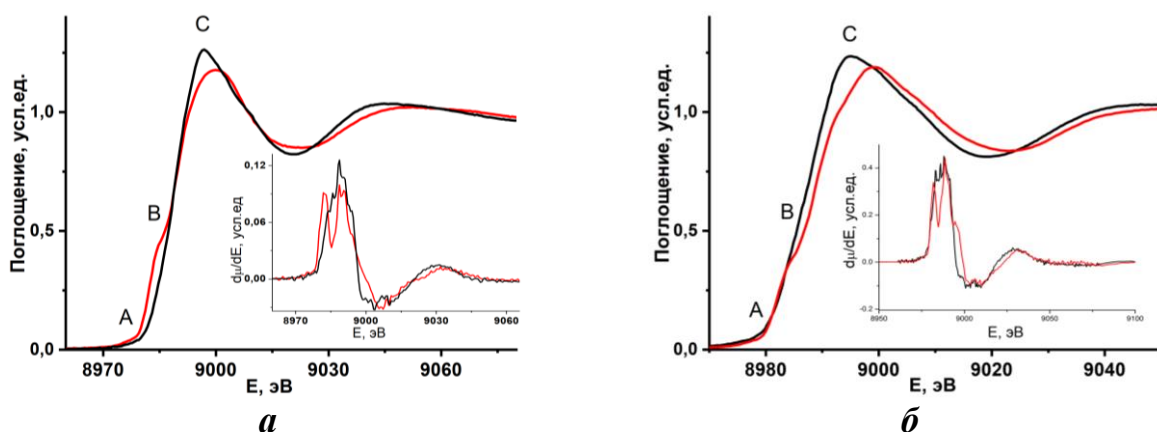
Рисунок 3.5 – Нормированные Cu К-края поглощения для соединений: 6 (черная линия) и 8 (красная линия) - (а), 7 (черная линия) и 9 (красная линия) - (б), соответствующие первые производные d\mu/dE показаны на вставках.
