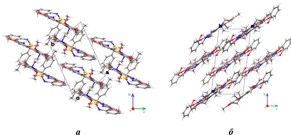
Рисунок 5.3 – Молекулярная структура комплексов 14 (a) и 15 (б)
