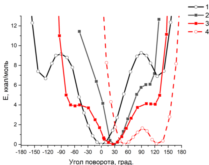
Рисунок 3.2 – Профили относительной энергии конформеров соединений 1 – 4 как функция торсионного угла поворота ароматического заместителя (хинолина, нафталина) относительно винилкетонового остова. Расчет выполнен на уровне B3LYP/6-311++G( d , p ) с оптимизацией геометрии при фиксированном торсионном угле.
