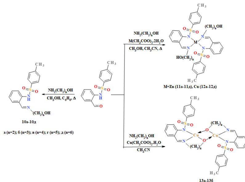
Схема 2.2 – Синтез оснований Шиффа 10a - 10д и их комплексов цинка(II) ( 11a - 11д ) и меди(II) ( 12a - 12д и 13a,136 )
