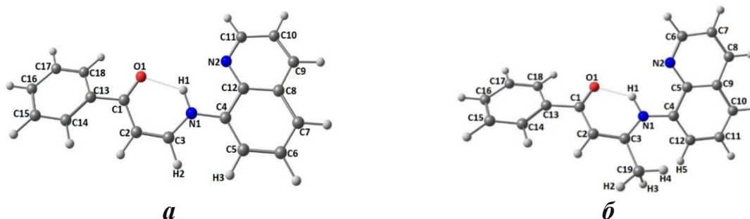
Рисунок 3.3 – Оптимизированные структуры 1 (а) и 2 (б)
