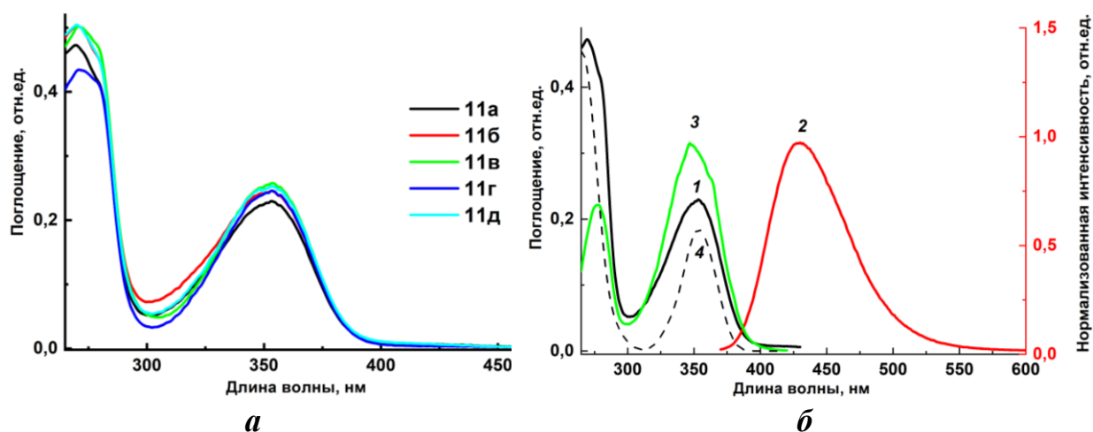
Рисунок 4.9 – ЭСП соединений 11a - 11d в ДМСО ( а ). ЭСП 11a в ультрафиолетовом диапазоне (1), излучения флуоресценции ( \lambda_{ex} = 350 нм) (2) и возбуждения флуоресценции ( \lambda_{obs} = 430 нм) (3) в ДМСО, пунктирная линия (4) показывает теоретически рассчитанный ЭСП ( б ).
