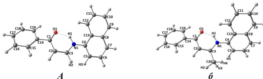
Рисунок 3.4 – Оптимизированные структуры 3 (а) и 4 (б)
