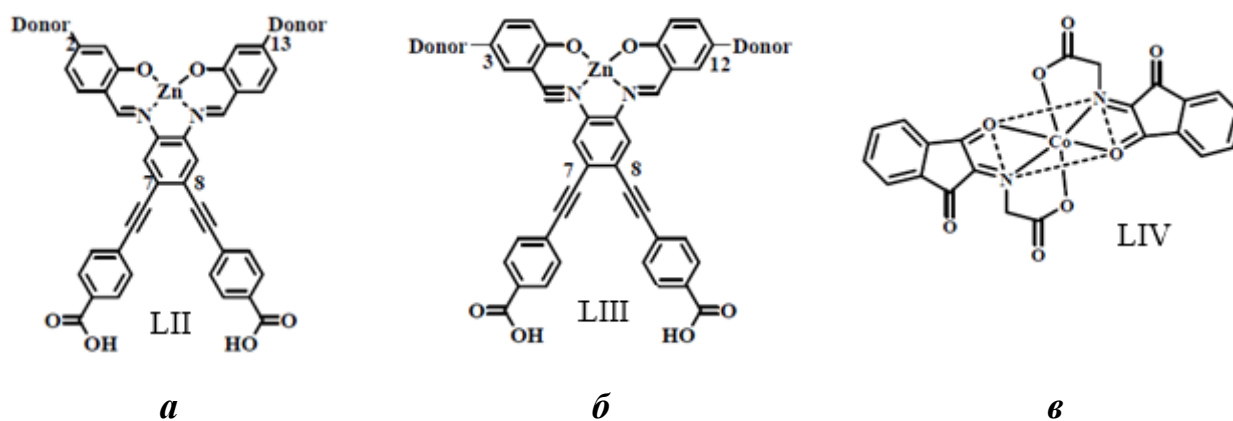
Рисунок 1.7 – Комплексы оснований Шиффа LII ( a ), LIII ( б ), LIV ( в )
