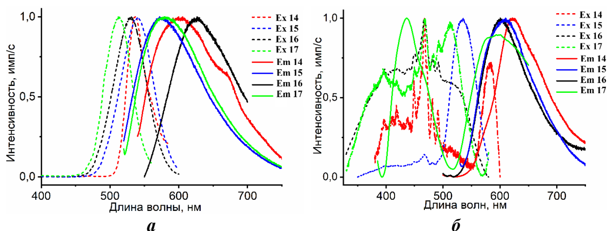
Рисунок 5.12 – Спектры возбуждения ( Ex ) и эмиссии ( Em ) комплексов 14 - 17 в хлористом метиле ( a ) и в твердом состоянии ( б )
