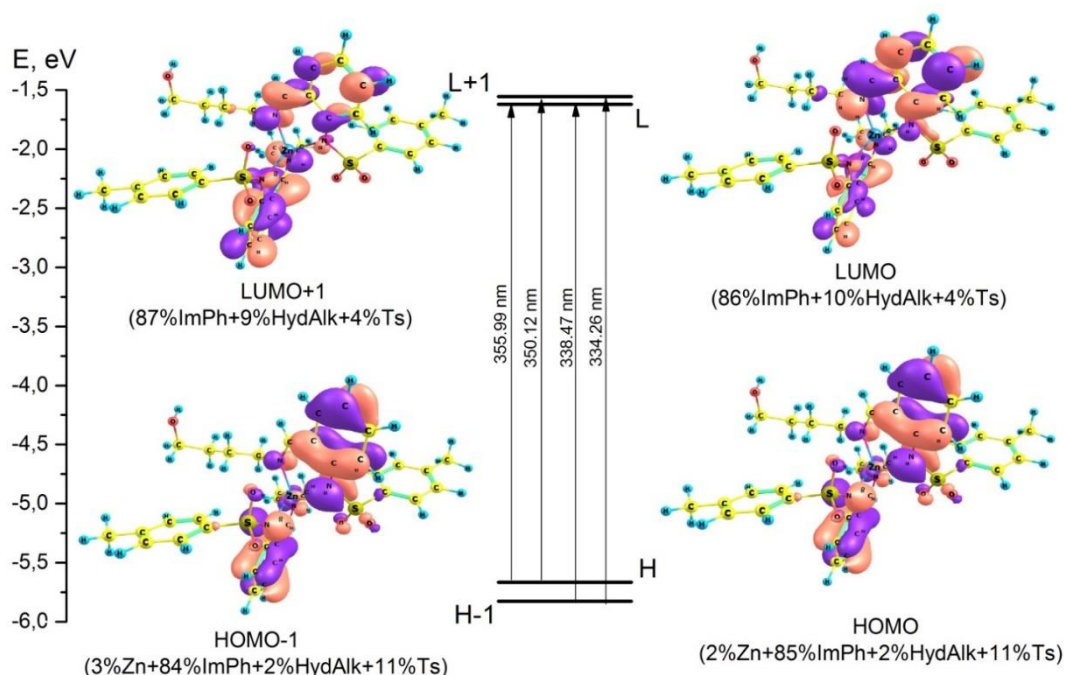
Рисунок Б.2 – Диаграмма энергетических уровней и изоповерхности пограничных молекулярных орбиталей для 11в и длины волн полученных электронных переходов, где иминометилфенильный (ImPh), тозильный (Ts), гидроксиалкильный (\text{CH}_2)_n\text{OH} (HydAlk) фрагменты.
