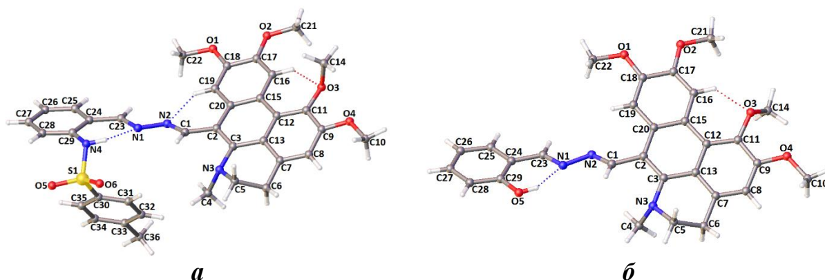
Рисунок 5.1 – Молекулярная структура комплексов 14 (а) и 15 (б)
