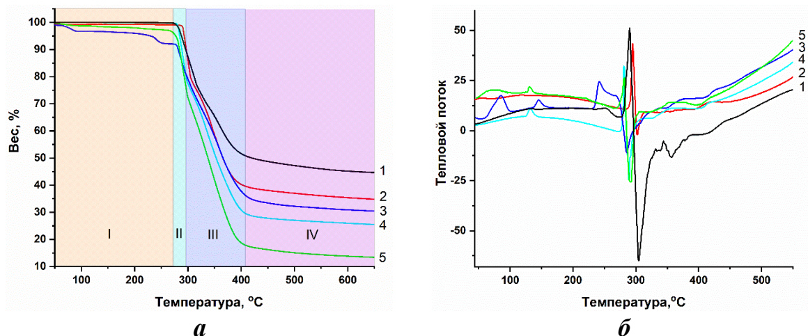
Рисунок 4.12 - Кривые ТГА ( а ) и ДСК ( б ) для 11а (1), 11б (2), 11в (3), 11г (4), 11д (5). I – область стабильности, II – область быстрой потери массы, III – возгонка с частичным разложением, IV – область стабильности продуктов разложения.
