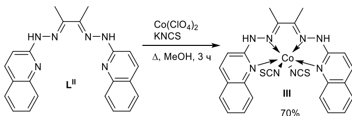
Схема 3 – Синтез соединения III
